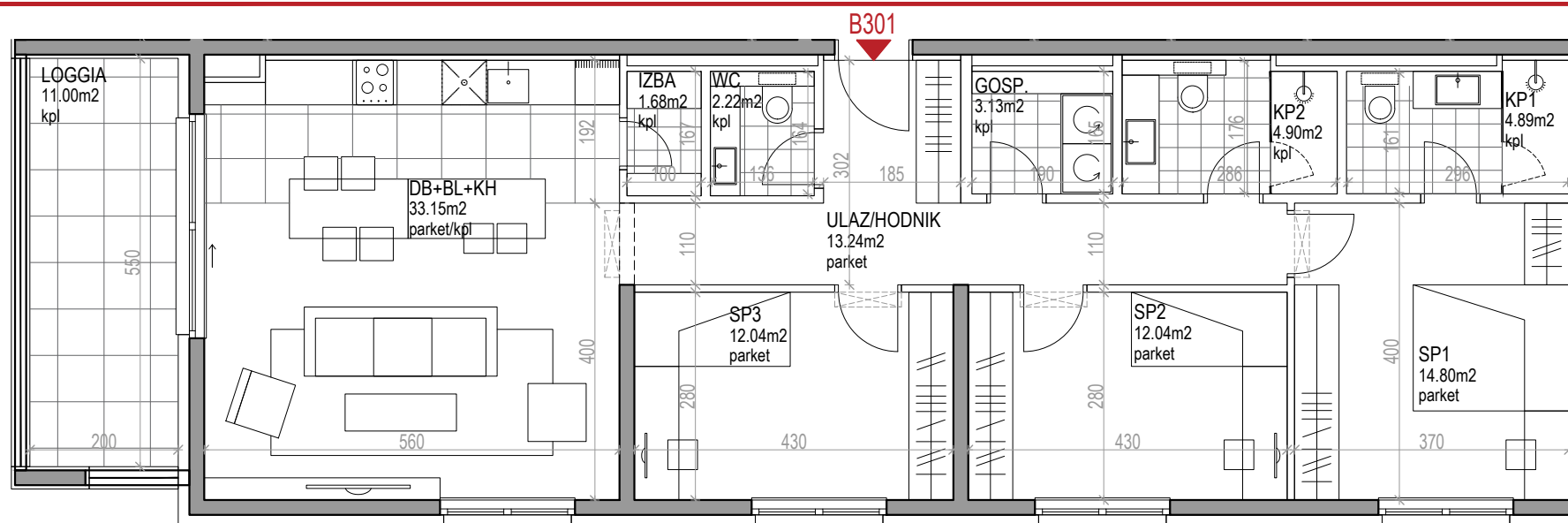
ČETVEROSOBAN STAN_3.KAT
